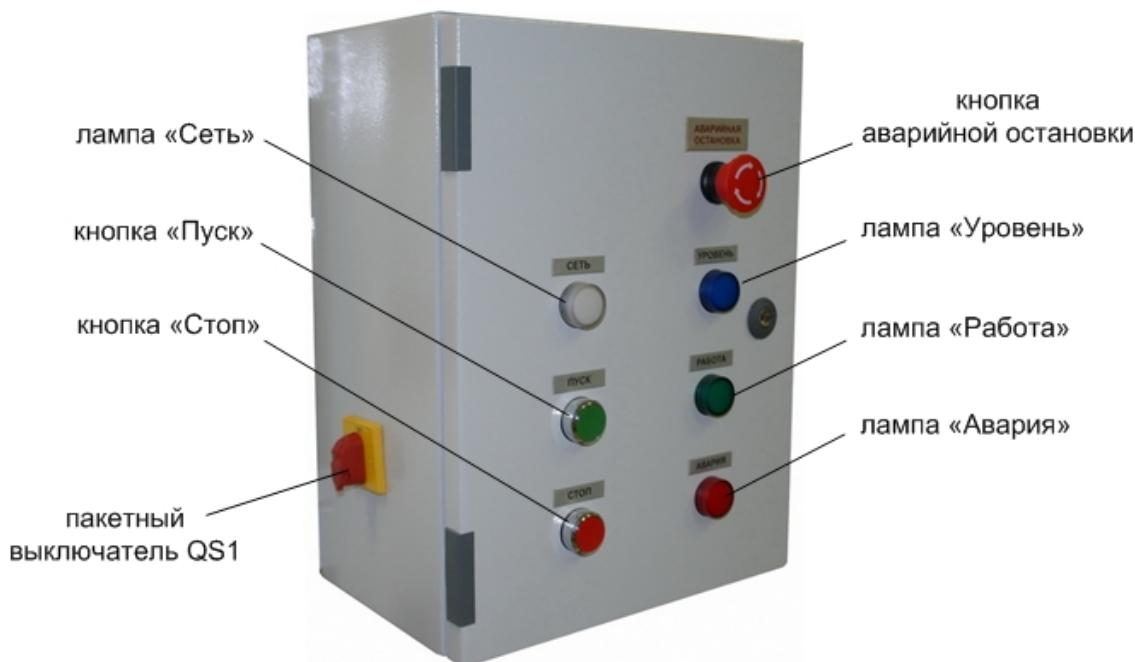
Рис.4 Блок управления.
