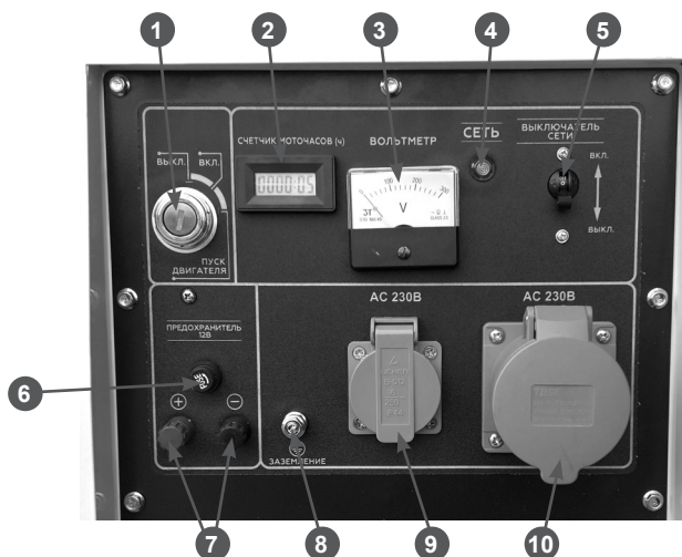
Рис. 3 Панель управления
